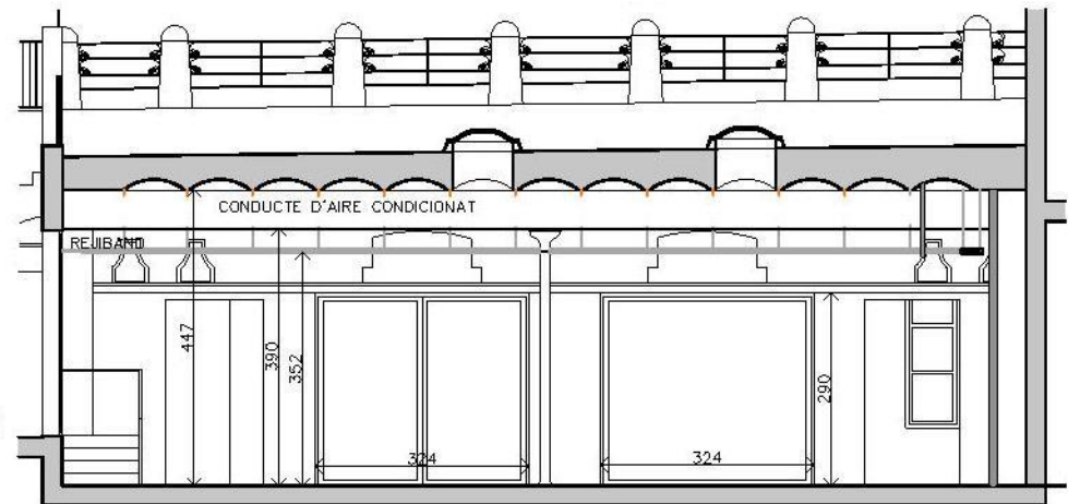
SECCIO INTERIOR. ESC 1/125
