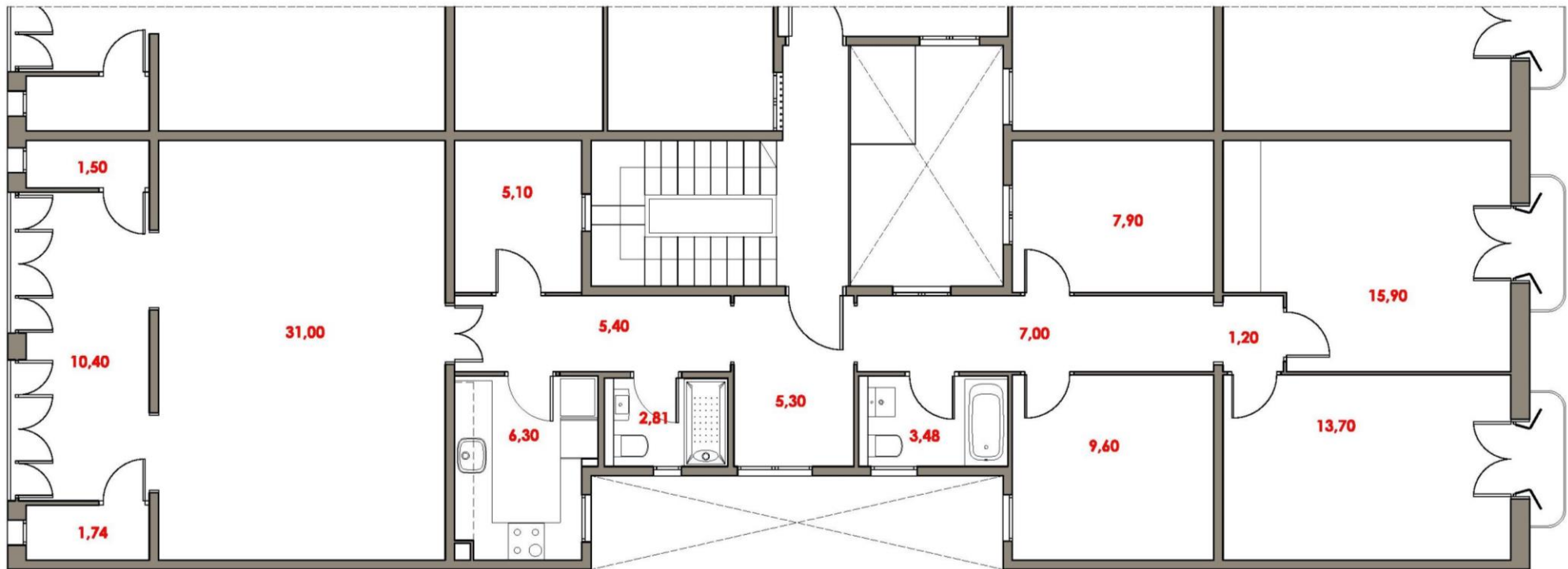
PLANTA E:1/50 SUPERFICIE UTIL: 128,33 m2
